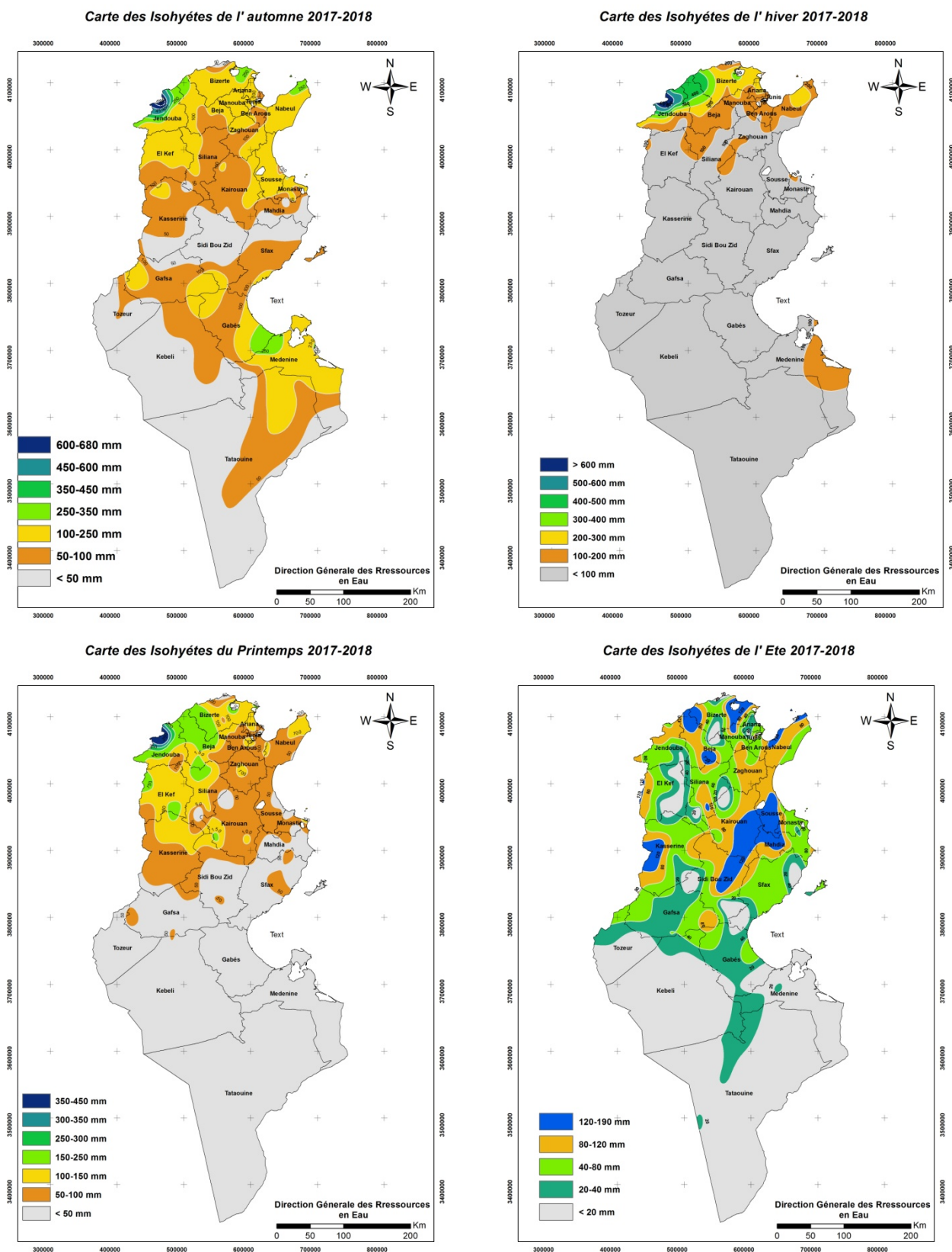
Figure 10: Isohyètes saisonnières de l'année 2017-2018
