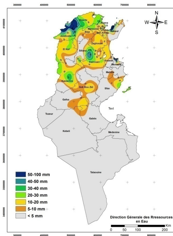
Carte des Isohyètes de Septembre 2017
