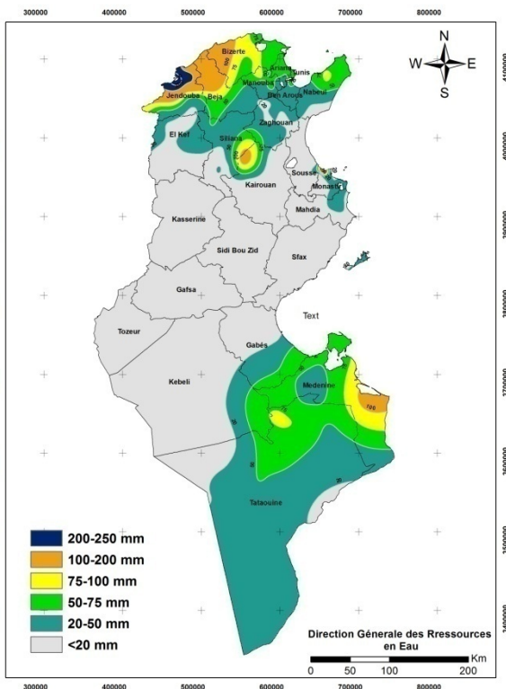
Carte des Isohyètes de Decembre 2017
