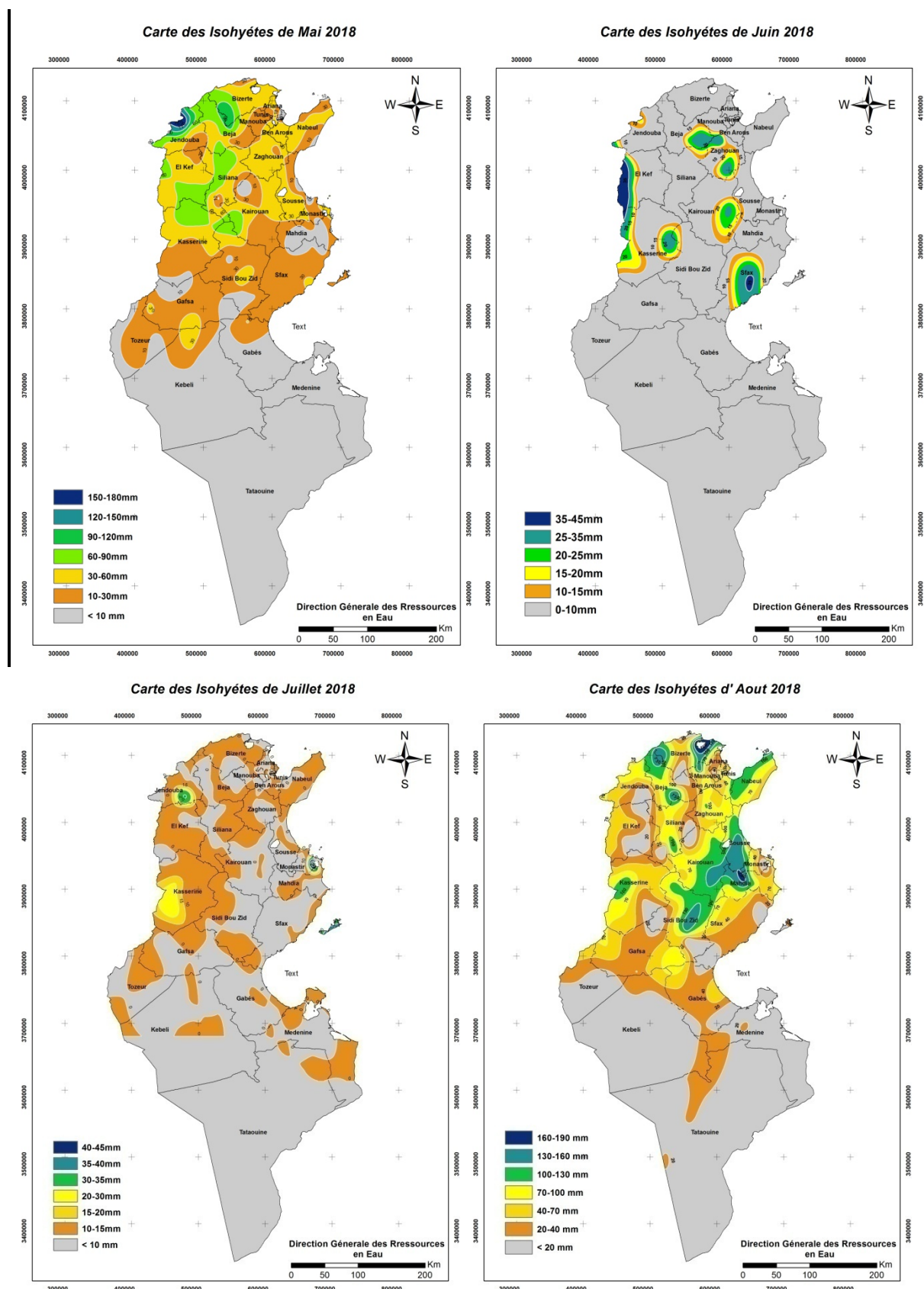
Figure 13: Isohyètes des pluies mensuelles des mois de (Mai, Juin Juil. et Août), année 2018
