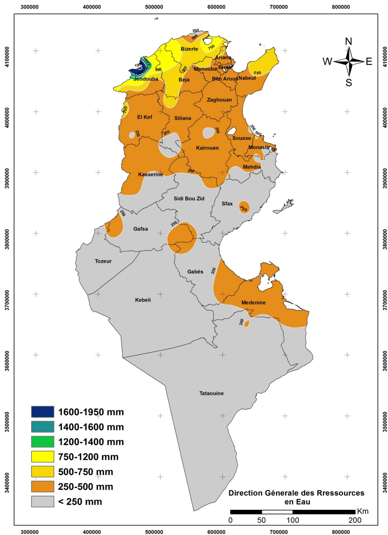
Figure 4 : Isohyètes de l'année 2017-2018
