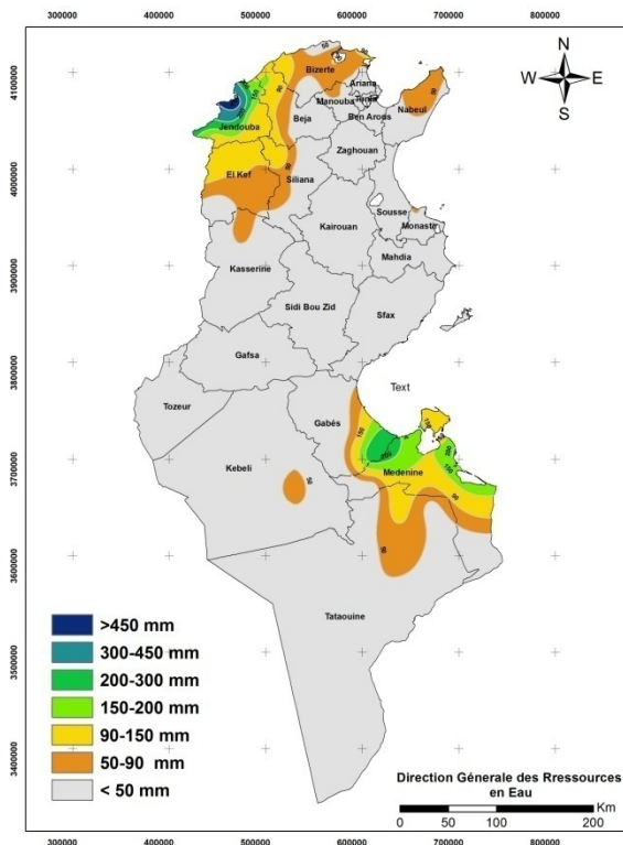
Carte des Isohyètes de Novembre 2017
