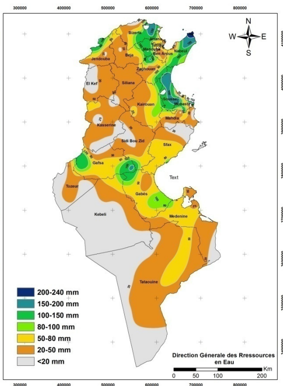
Carte des Isohyètes d'Octobre 2017
