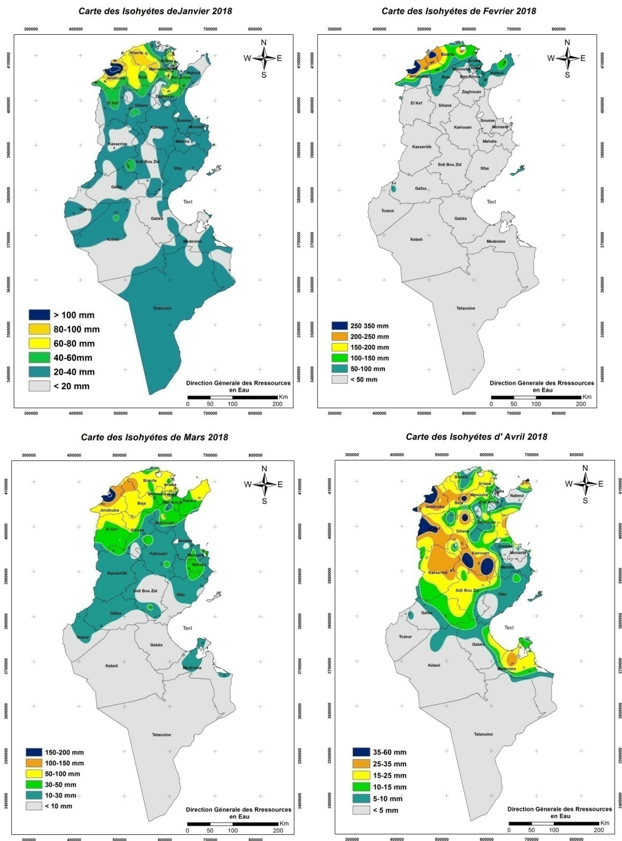
Figure 12 : Isohyètes des pluies mensuelles des mois de (Janv., Fév., Mars et Avril), année 2018
